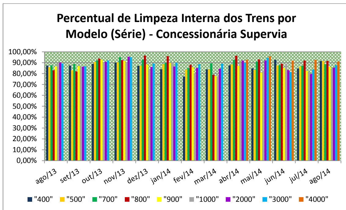
Gráfico 3-150 Supervia - Limpeza Interna - Trens Inspeccionados
