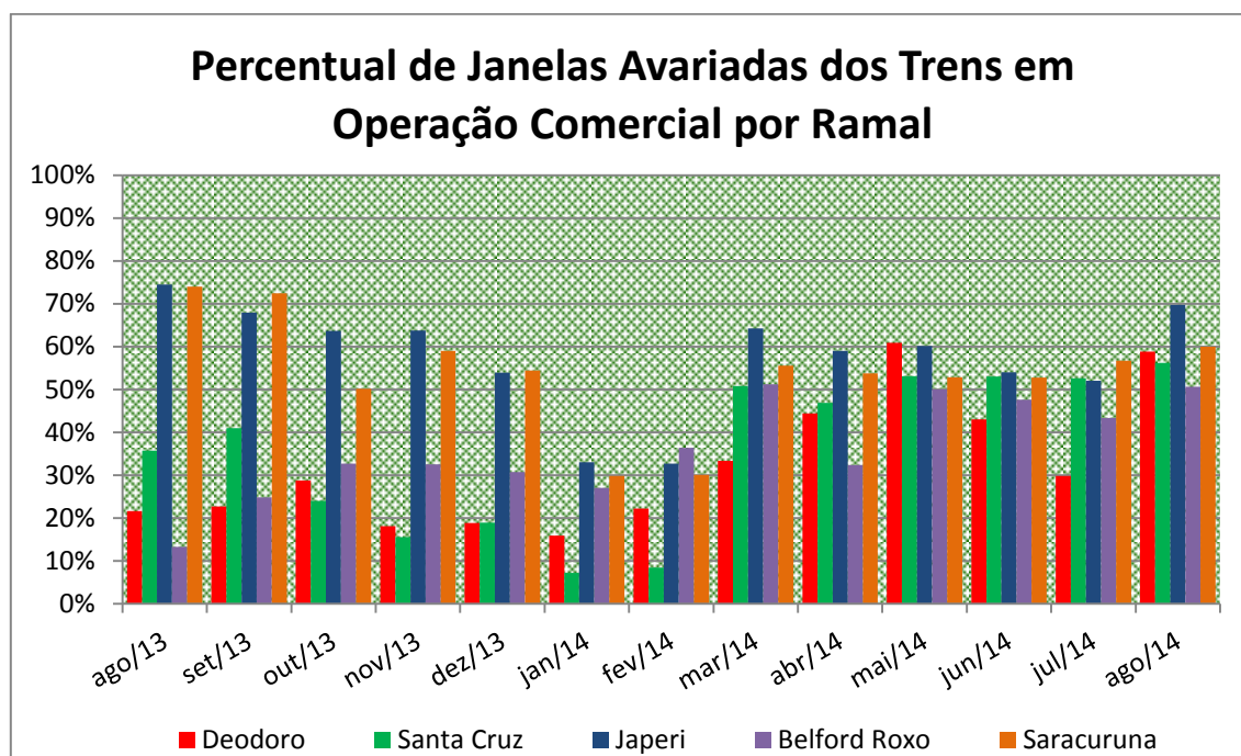
Gráfico 3-142 Supervia - Janelas - Por Ramal
