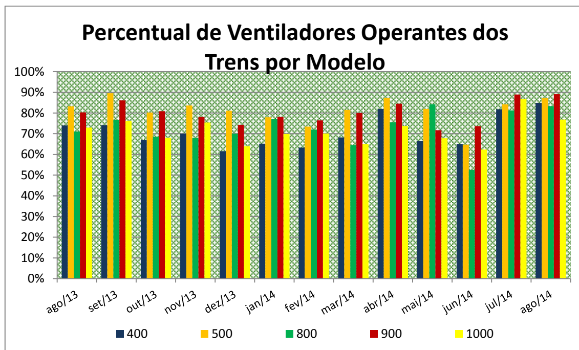
Gráfico 3-163 Supervia - Ventiladores - Por Série
