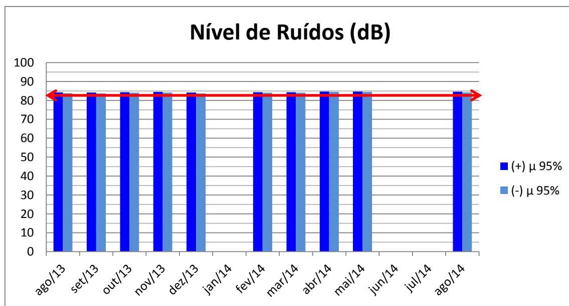
Gráfico 3-69 Metrô Rio – Aferição de Ruídos
